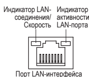
Индикатор LAN-соединения/Скорость
