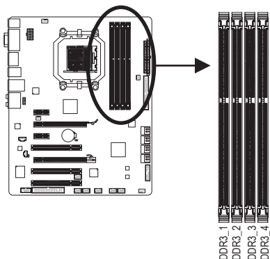
► Dualchannel-Speicherkonfigurationstabelle
