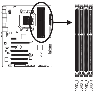
► Tabella di configurazione memoria Dual Channel
