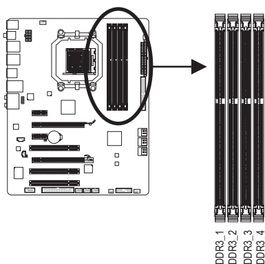
► Dualchannel-Speicherkonfigurationstabelle
