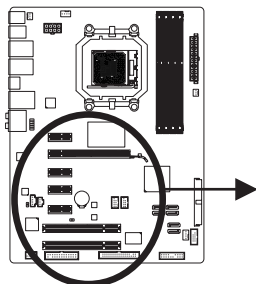
Разъем порта PCI Express x1
