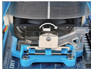
Fase 4: Ruotare l'impugnatura della cappa dal lato sinistro al lato destro (come mostrato dall'immagine) per fissarlo. (Fare riferimento al manuale del dissipatore di calore CPU per istruzioni su come installare il dissipatore.)
