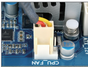
Fase 5: Infine, collegare il connettore d'alimentazione del dissipatore di calore CPU al connettore ventolina CPU (CPU_FAN) della scheda madre.
