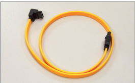
Conecte el extremo con forma de L del cable SATA de 3 Gb/s a la unidad de disco duro SATA.
