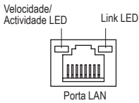
Velocidade/Actividade LED:
