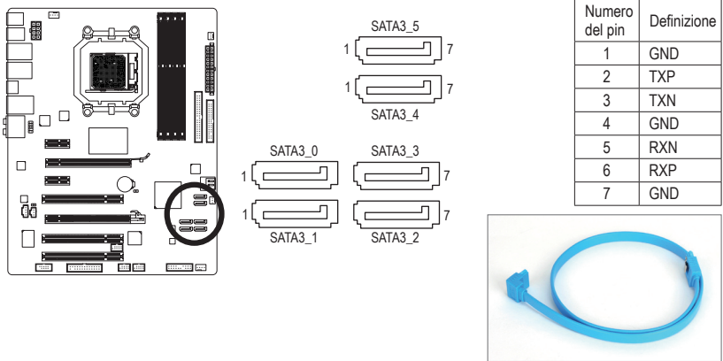
Collegare il terminale a forma di L del cavo SATA al disco rigido SATA.
