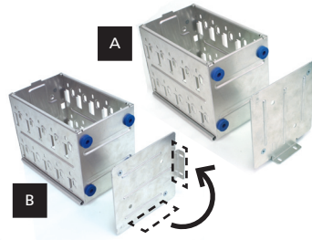
4-9.2 將可移動式硬碟架的免工具固定扣向下壓並予以解開
