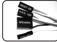
基本開關燈訊控制線材
