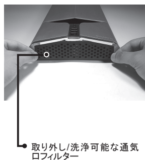
d) 底部パネル
